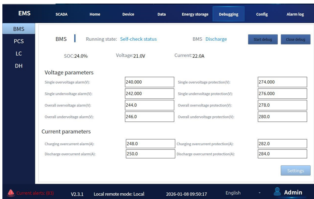
Abbildung 7.8-1 BMS
