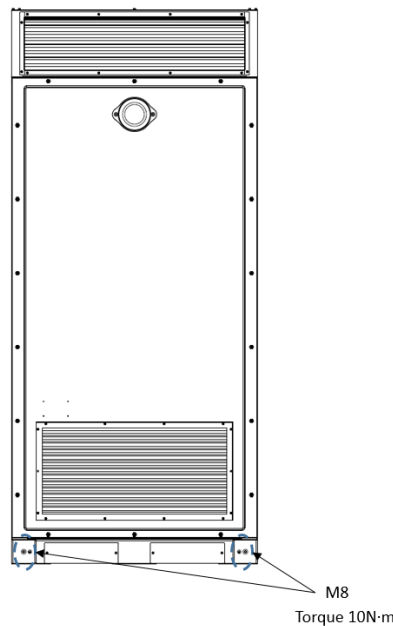
Abbildung 5.2-1 Externe Anschlüsse für die Erdung
