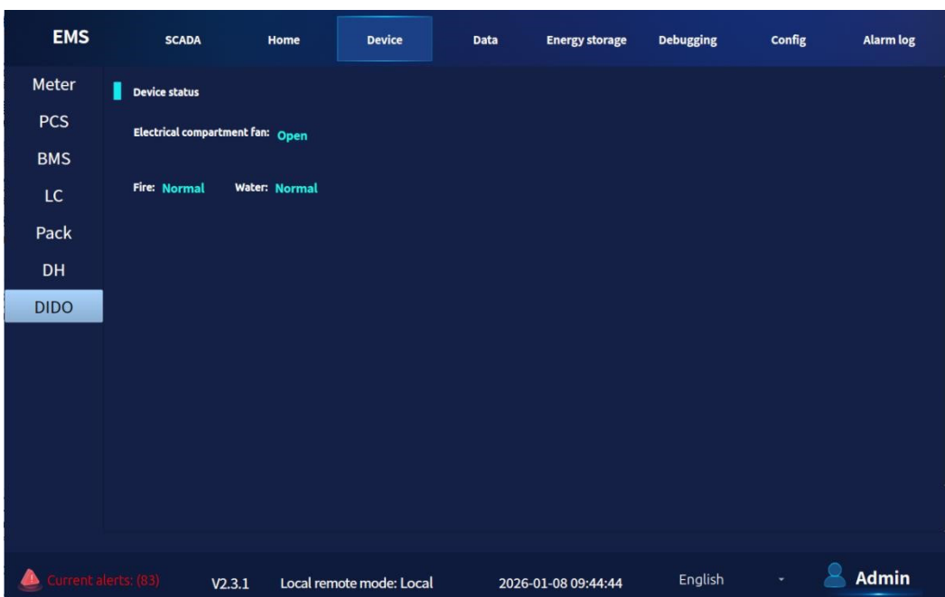
Abbildung 7.5-7 DIDO Interface
