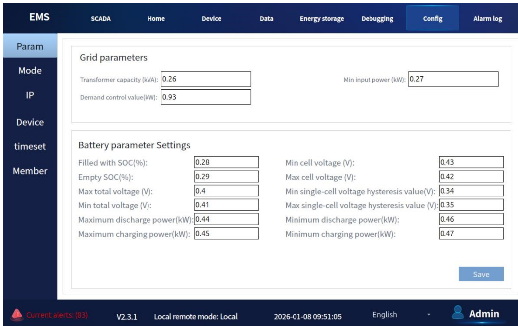
Abbildung 7.9-1 Systemparameter
