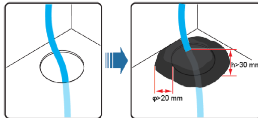
Abbildung 5.3-5 Darstellung der Versiegelung mit Brandschutzmasse
