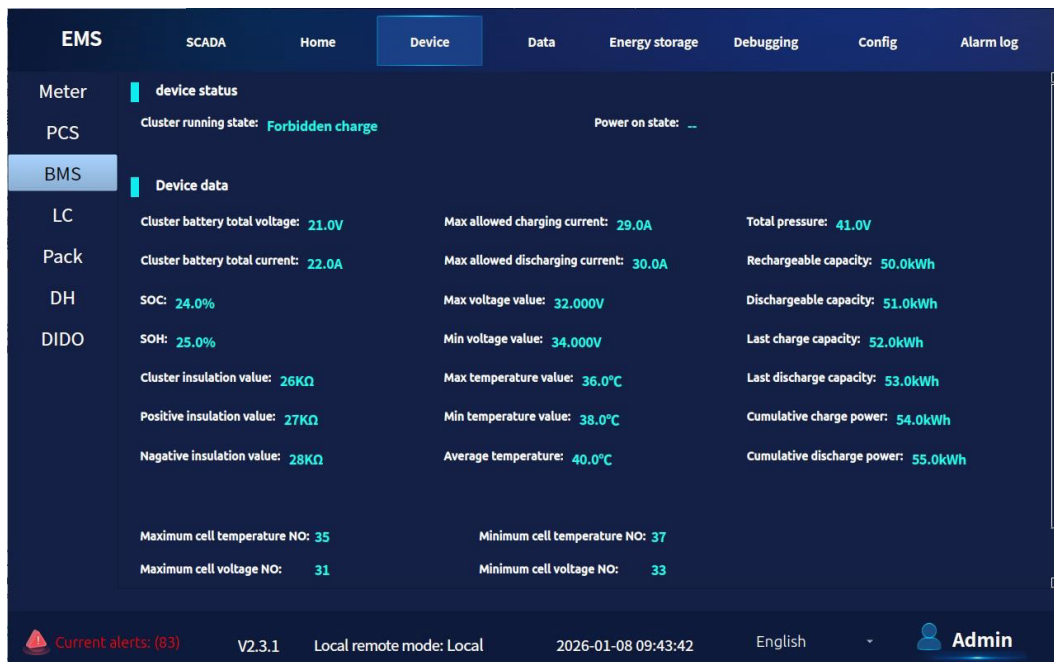
Abbildung 7.5-3 BMS Interface
